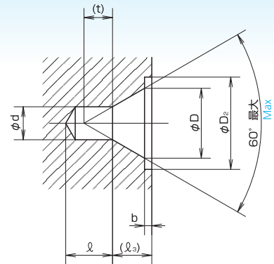
C形 Type C
