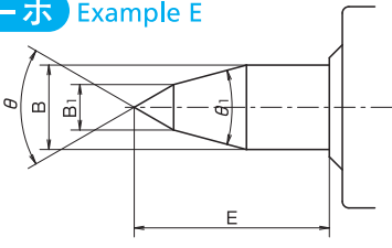
インセンター(逆センター) Inverted center
