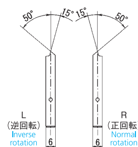
J 矢視図 J arrow diagram
