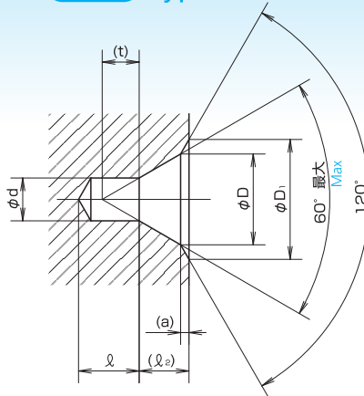
B形 Type B
