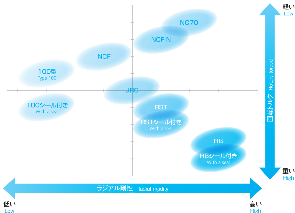
● ローリングセンター シャンク別選定表 Table for selecting a rolling center model with shanks
