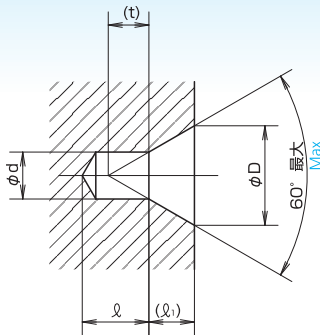
A形 Type A
