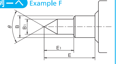
インセンター(逆センター) Inverted center
